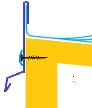
Obr. 9 - Závětná lišta
