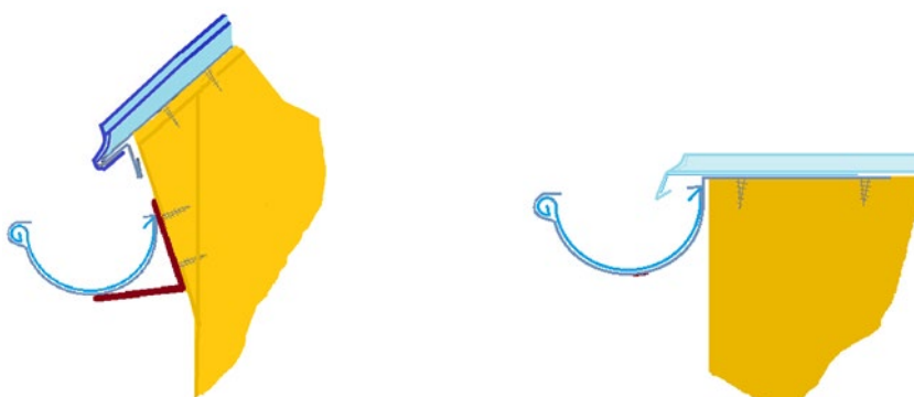
Obr. 7 - Zapravení u okapu
