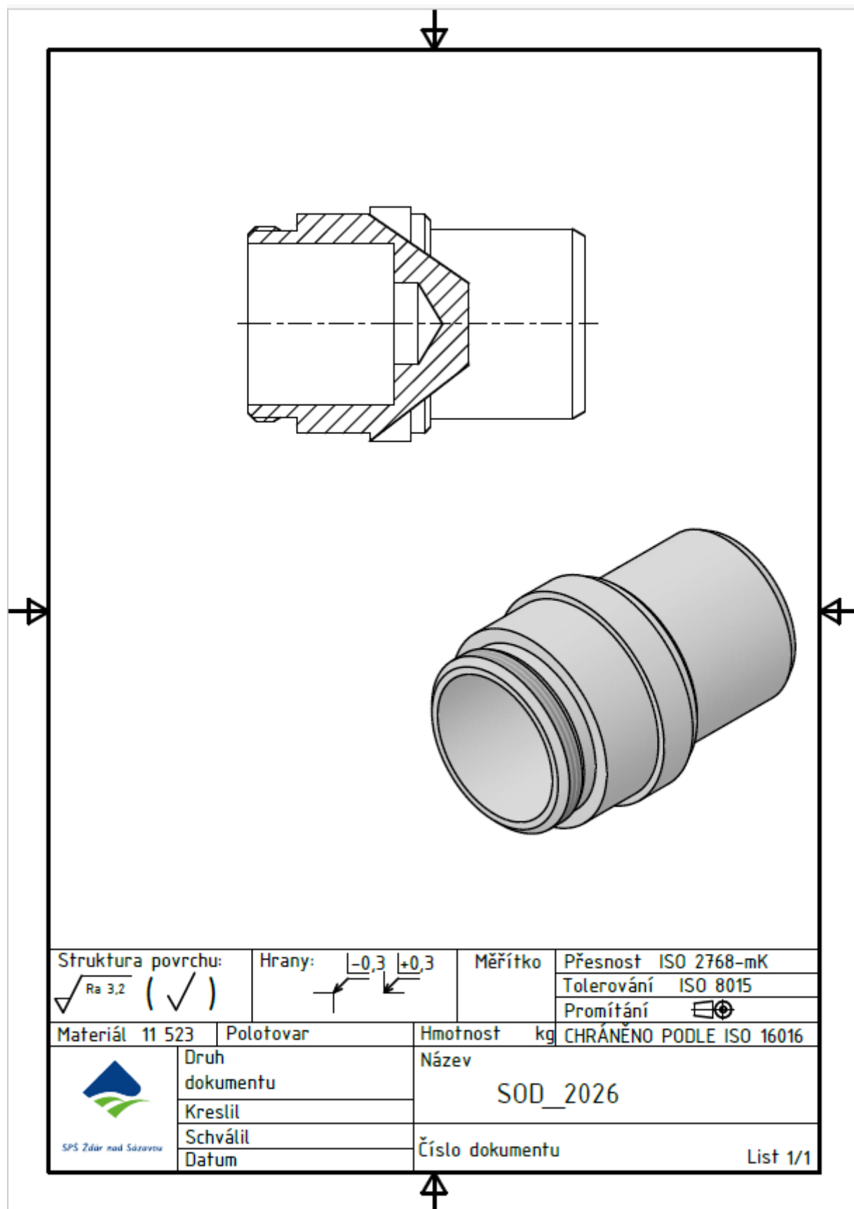
Příloha č. 1 – výkres
