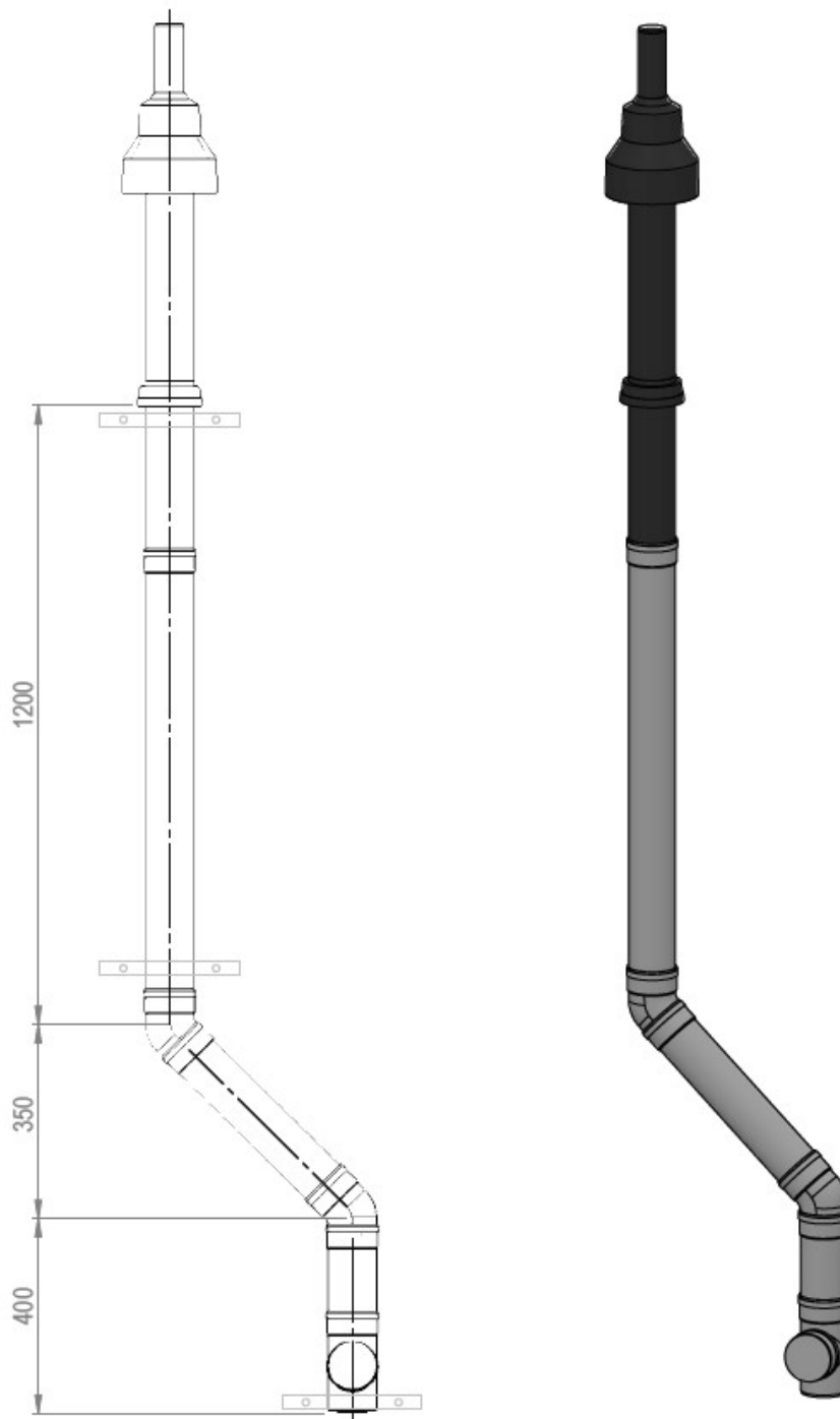
Obrázek 4, výkresová dokumentace pro montáž spalinové cesty Almeva
